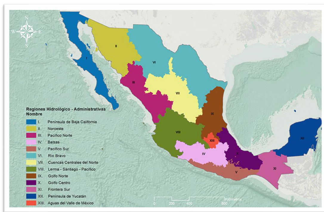
Mapa 1. Las 13 Regiones Hidrológico Administrativas en que se divide el territorio nacional. Tomado de Semarnat (2020).
