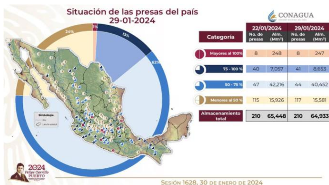
Imagen 2. Situación de presas al 29 de enero de 2024. Tomado de Redacción (2024).
